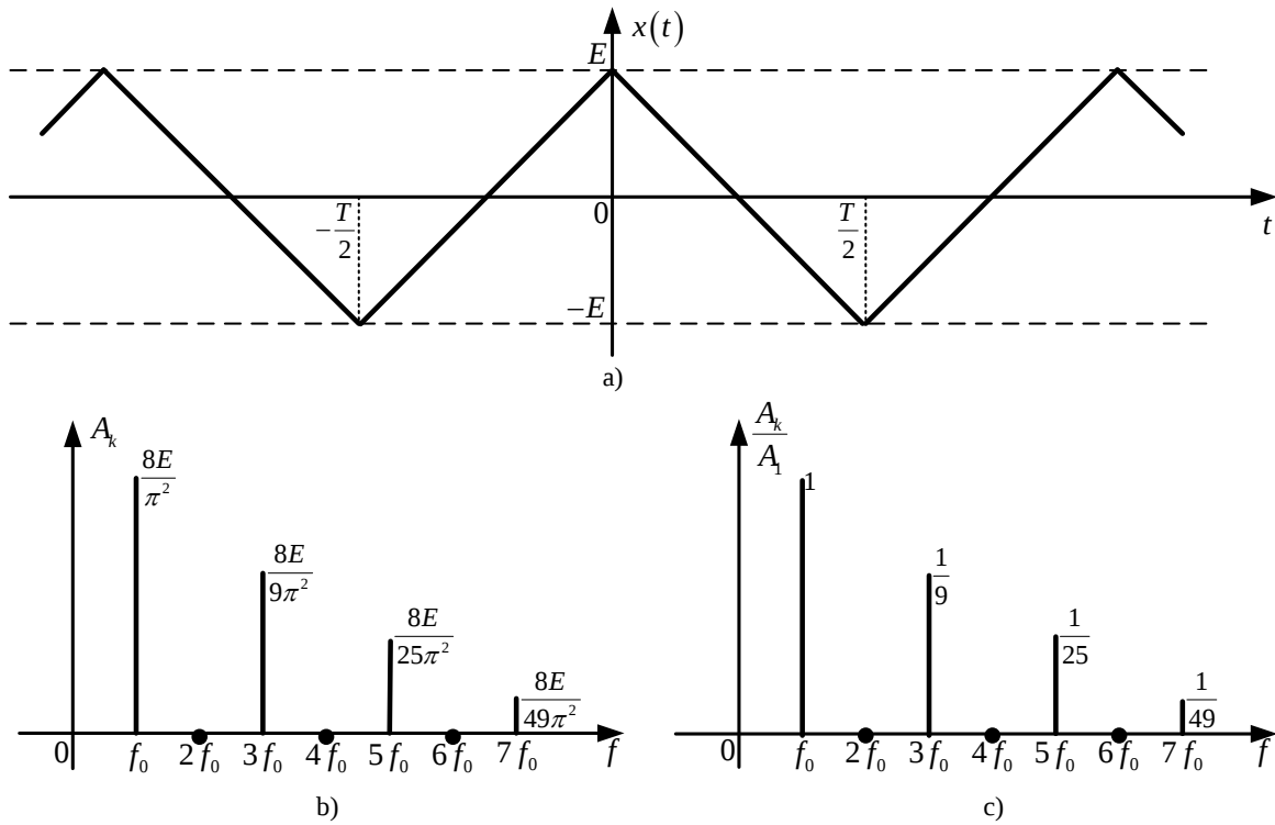
Figura 3. a) Reprezentarea în timp a semnalului triunghiular; b) Spectrul de amplitudini pentru semnalul triunghiular; c) Spectrul de amplitudini normat pentru semnalul triunghiular
