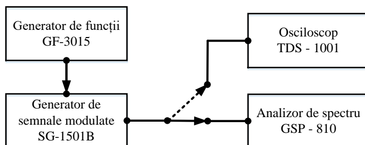
Figura 6. Schema de măsură folosită în lucrare
