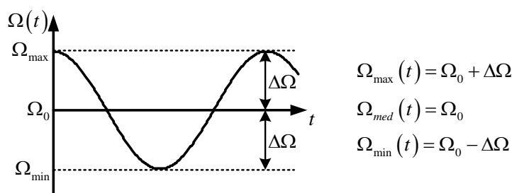
Figura 1. Reprezentarea grafică a frecvențelor instantanee pentru un semnal MF cu purtător armonic și semnal modulator armonic
