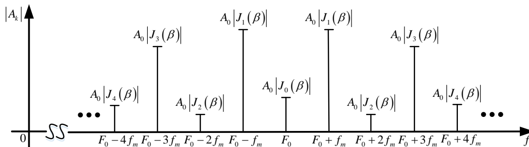
Figura 4. Diagrama spectrală de amplitudine pentru un semnal MF cu purtător armonic și semnal purtător armonic
